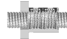
JTi Reihe: Präzisions-Kugelgewindetrieb in Zollauführung, Mutter m. weichem Flansch, Genauigkeitsklasse IT 1: 6µm, IT 3: 12µm, IT5: 23µm, IT7: 52µm Steigungsfehler
