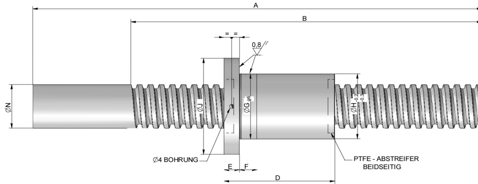
JTi Reihe: Präzisions-Kugelgewindetrieb in Zollauführung, Mutter m. weichem Flansch, Genauigkeitsklasse IT 1: 6µm, IT 3: 12µm, IT5: 23µm, IT7: 52µm Steigungsfehler
